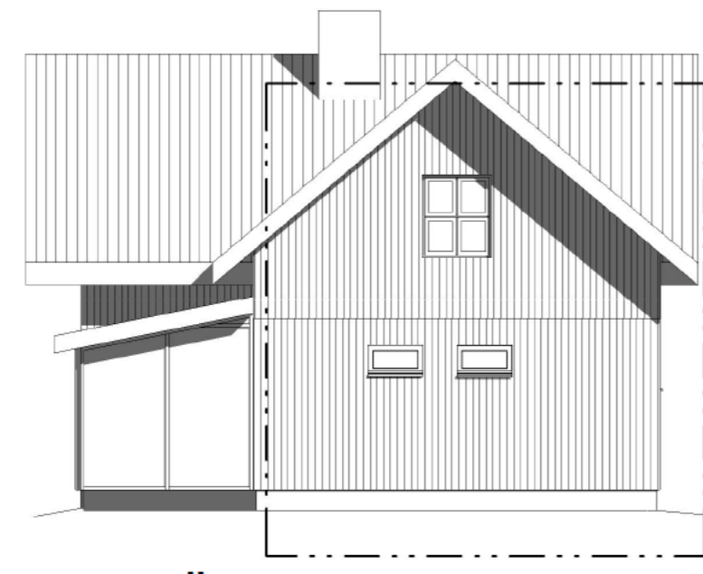
2 ITÄ 1 : 100 LAAJENNUS
