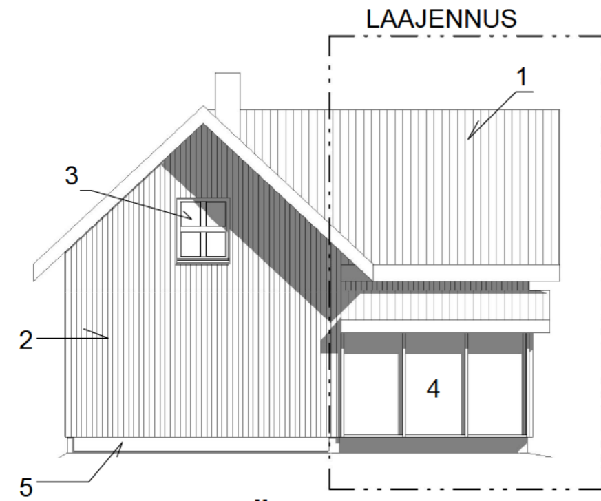
1 ETELÄ 1 : 100 LAAJENNUS
