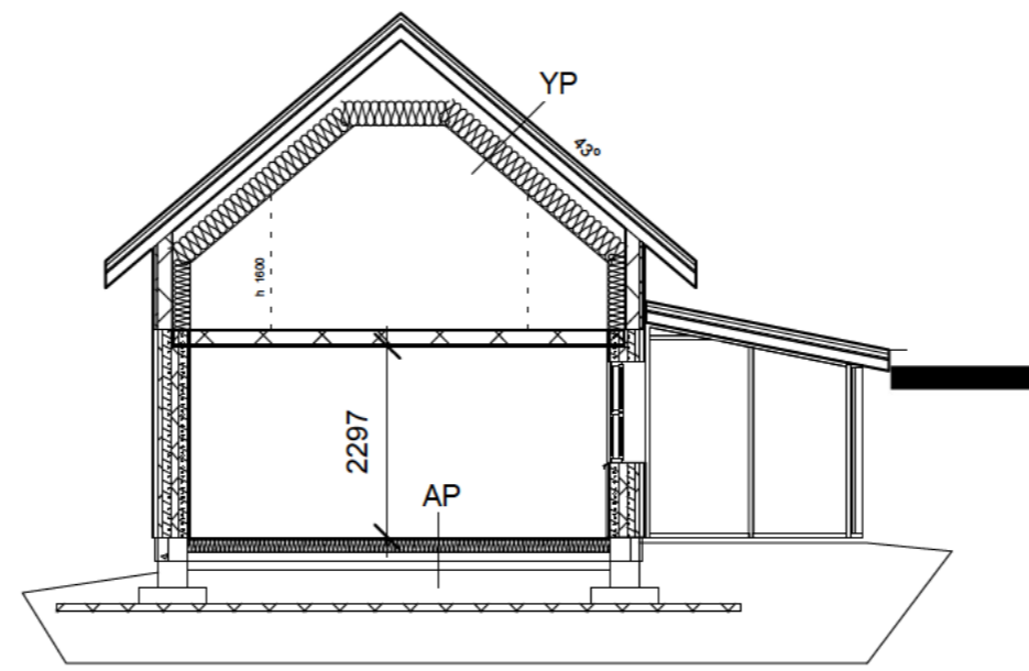
5 LEIKKAUS 1 : 100
