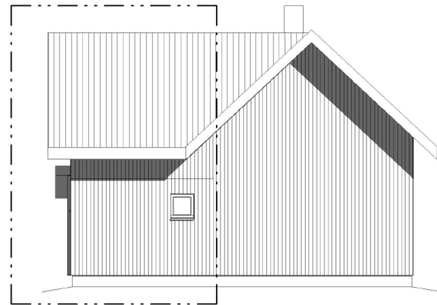
4 POHJOINEN 1 : 100
